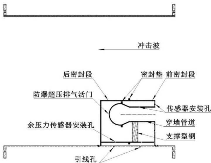
图 B. 4 防爆波超压排气活门固定方式示意图
