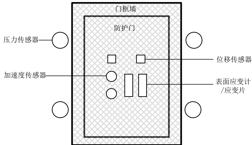
(b) 传感器布置图
