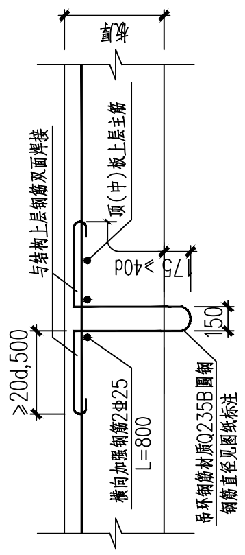
顶板吊环详图
