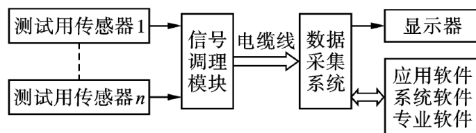
图C.2 抗力性能测试系统工作原理示意图
